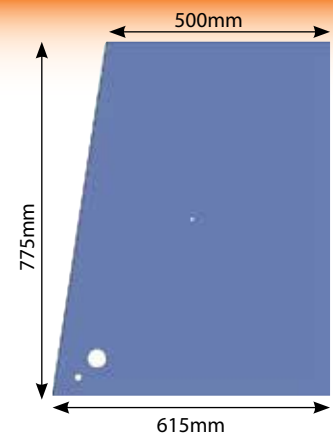
Glass 300 Door Top
