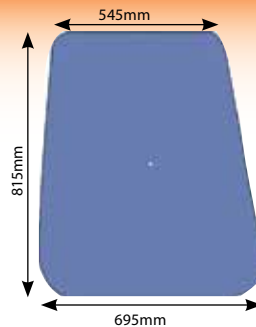
4582 Glass Ford Q Cab Upper Door
